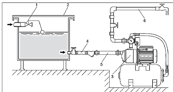
Montaj hidrofor – vas tampon 1 - Robinet plutitor 2 – Vas tampon 3 – Hidrofor 4 – Supapa de sens 5 – Conducta de aspiratie 6 – Conducta de refulare
